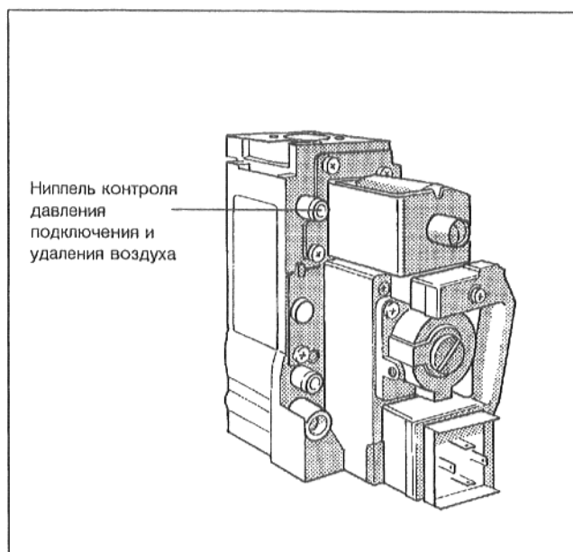
Рис. 15: Арматура газовой горелки "Honeywell" VR 4601
