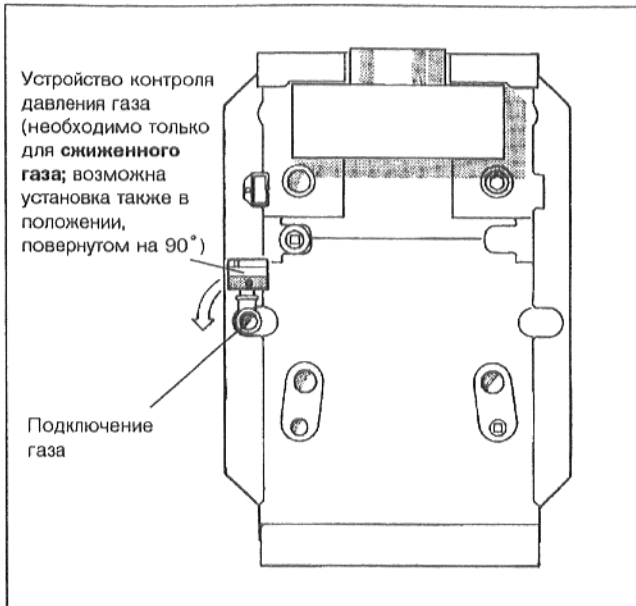
Рис. 13: Подключение газа
