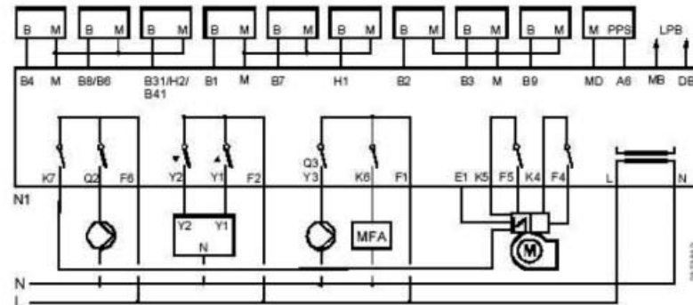
Соединения для модуляционной горелки
